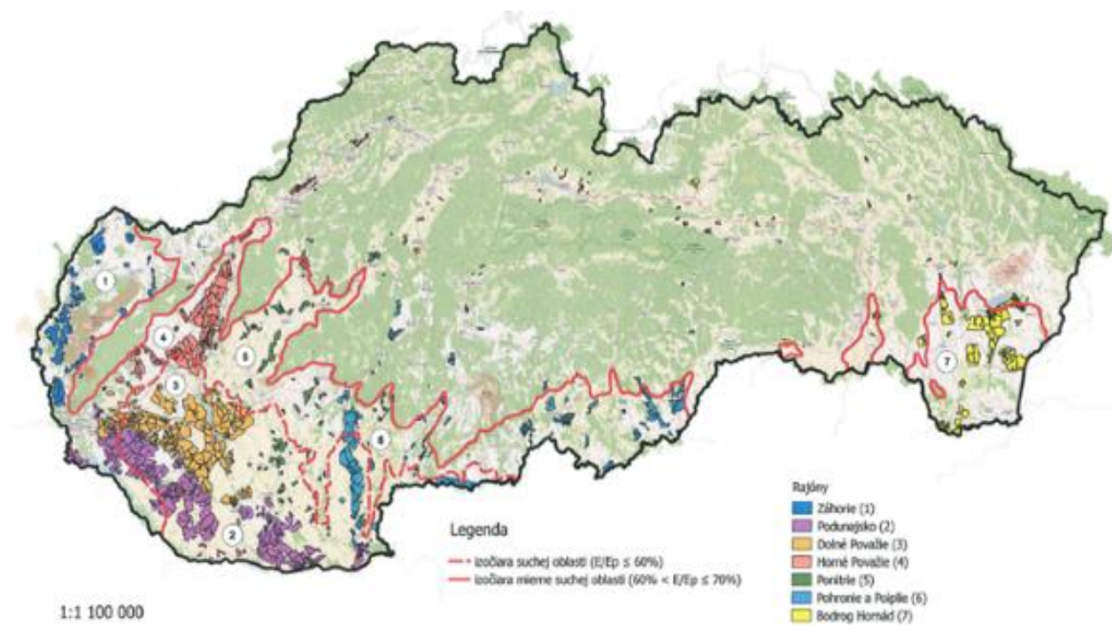
Mapa 5 Rajonizácia závlahových sústav na Slovensku v správe Hydromeliorácie, š. p.
